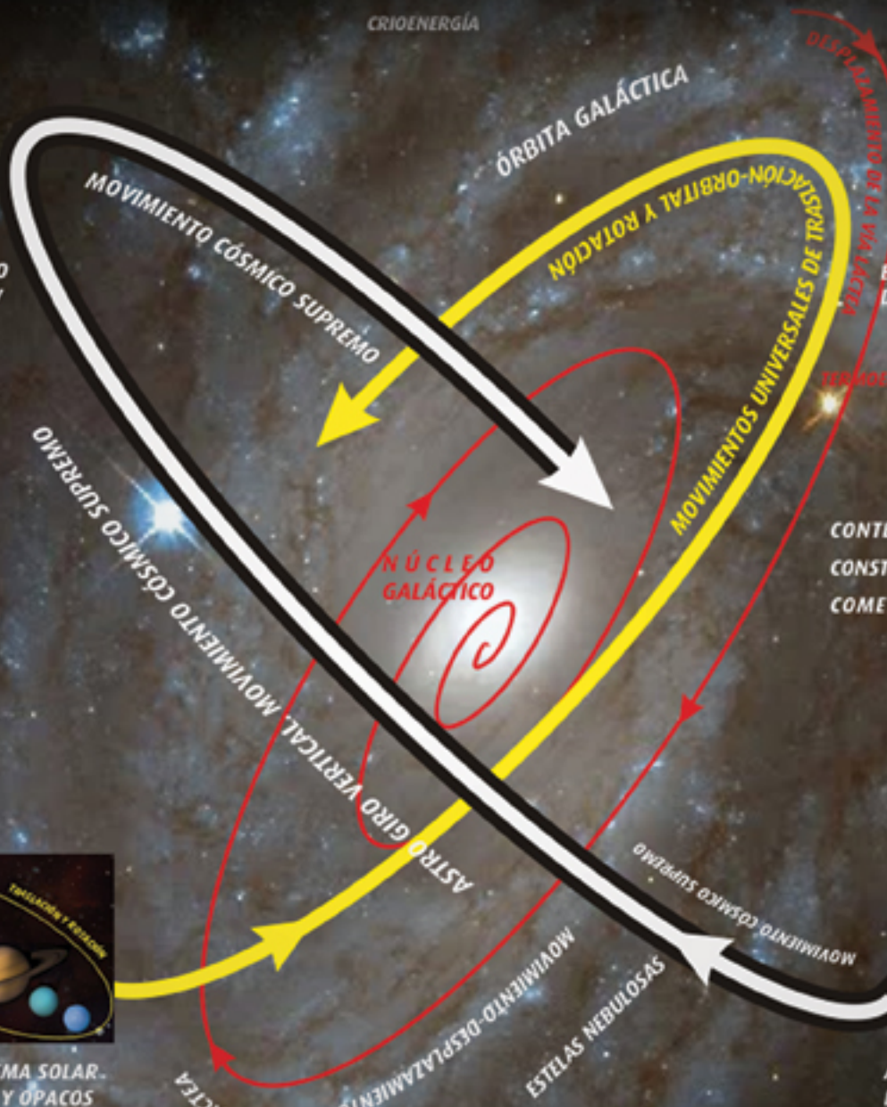
NACIMIENTO DEL UNIVERSO COORDINACIÓN VVV Y AGV
